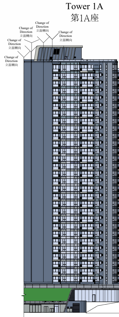
ELEVATION PLAN 2 立面圖 2
