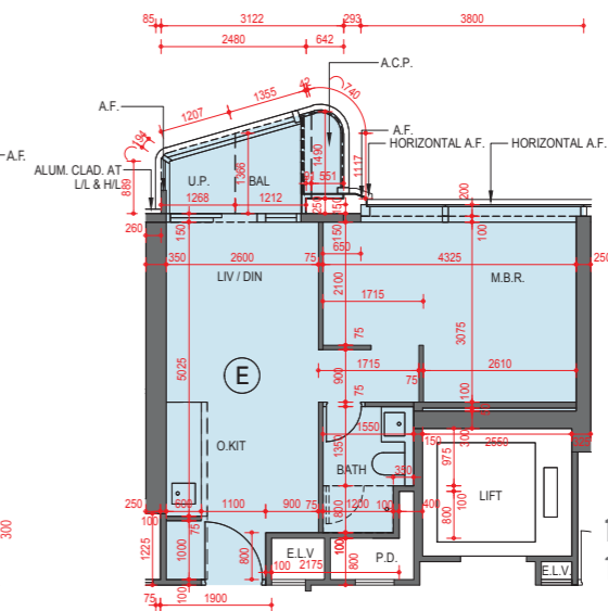
18/F Part Plan of Flat E 18樓E單位部分平面圖
