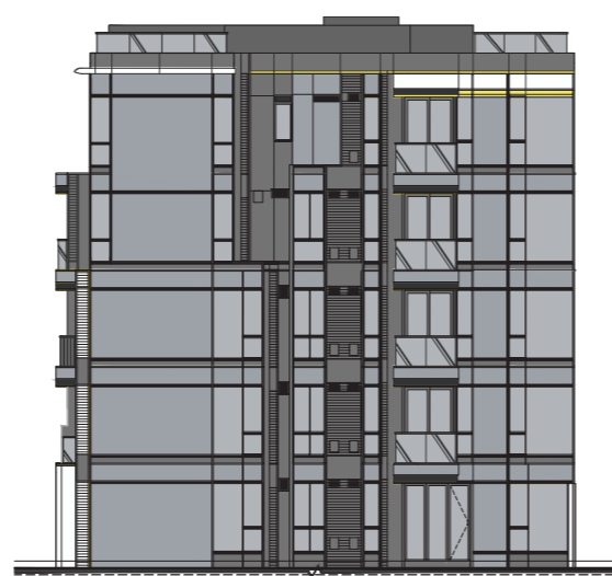
Elevation 2 立面圖2
