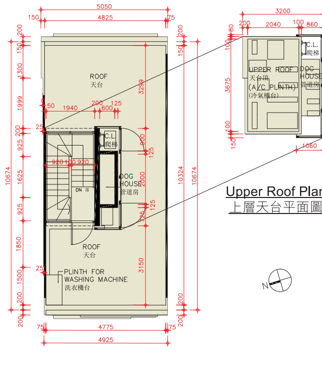
Roof Plan 天台平面圖
