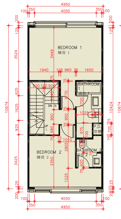
2/F Plan 2樓平面圖
