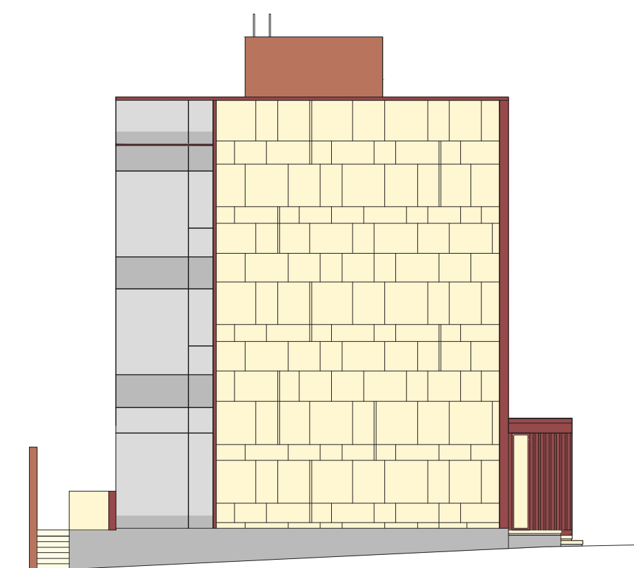
側立面圖 SIDE ELEVATION
