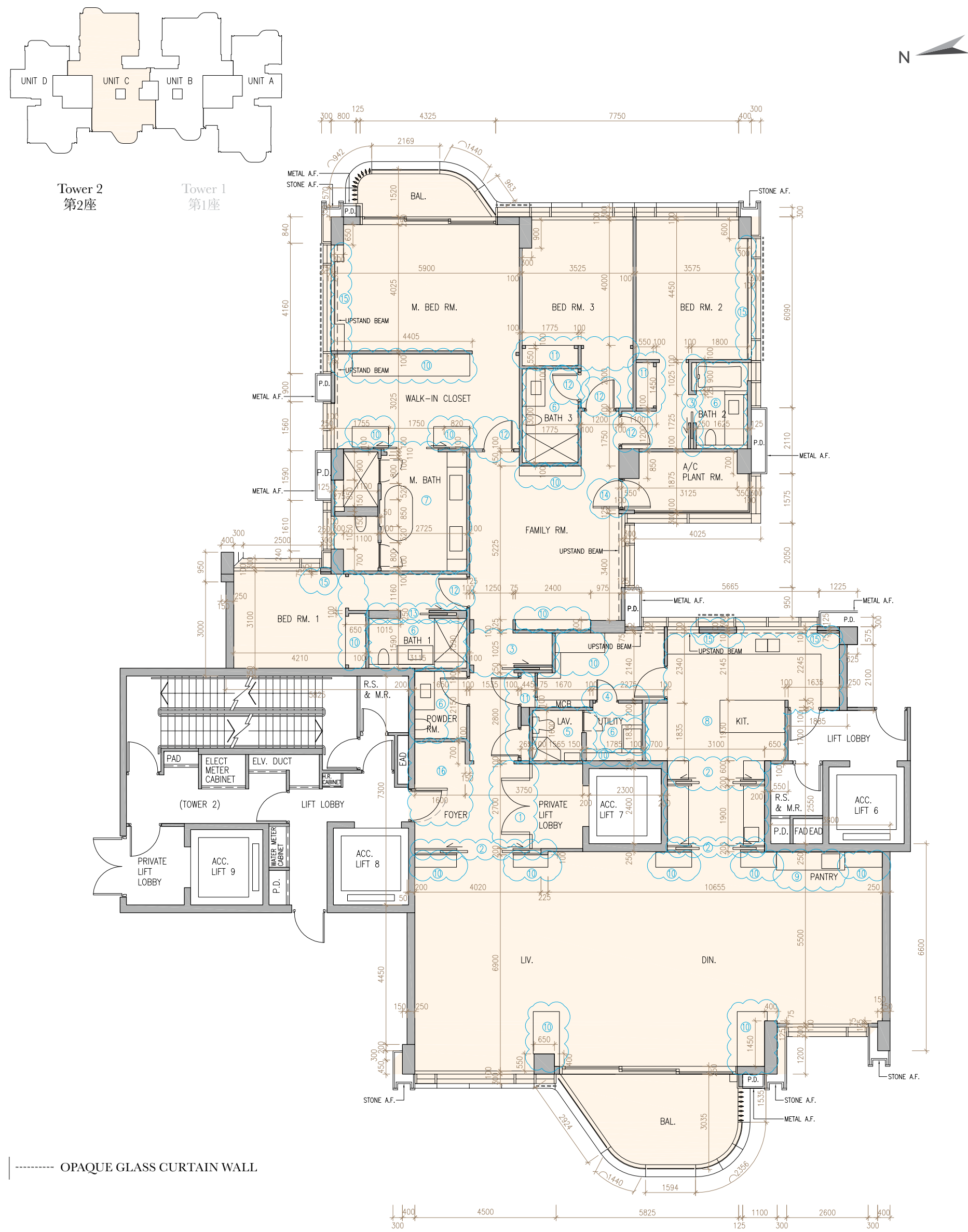
UNIT C 16/F FLOOR PLAN SHOWING LATEST LAYOUT C 單位 16樓現狀樓面平面圖
