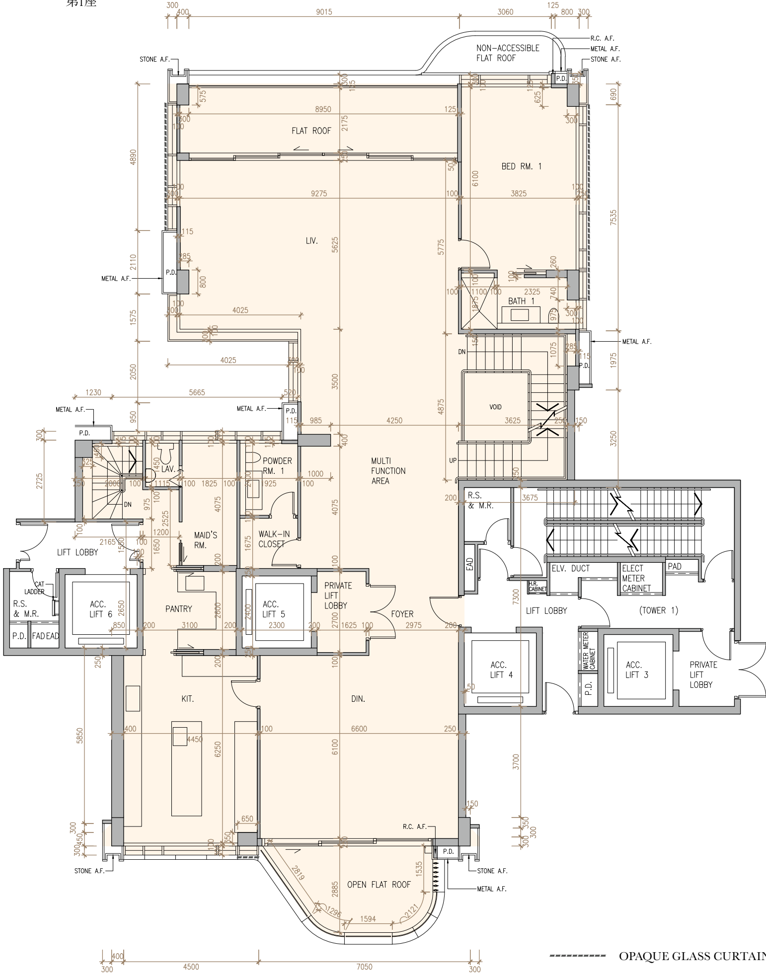
PENTHOUSE B 19/F FLOOR PLAN 頂層單位 B 19樓樓面平面圖
